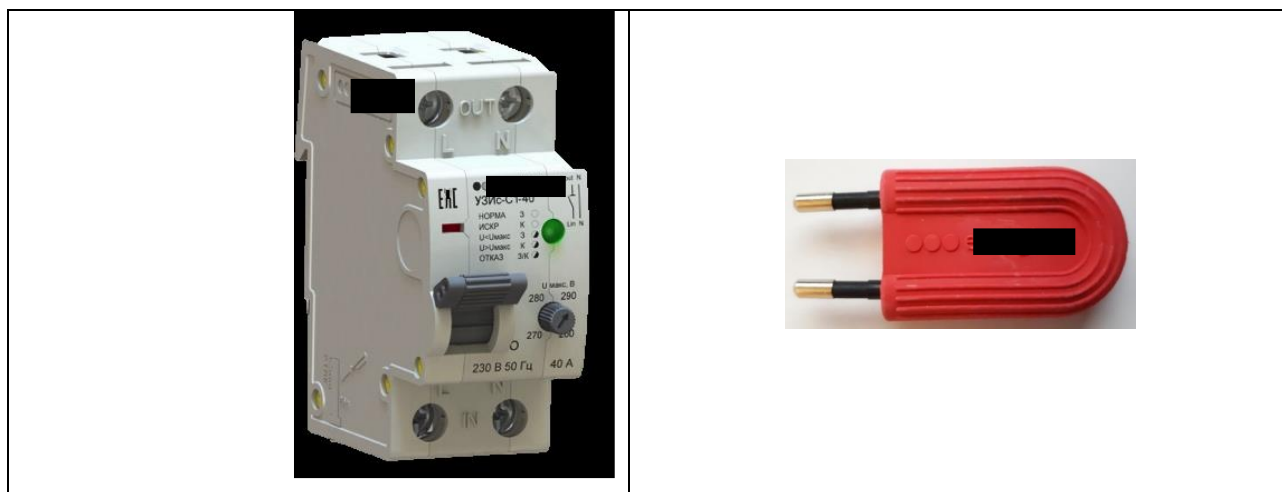
Рисунок 10. Пример УЗДП в комплекте со средством контроля зоны функционирования
